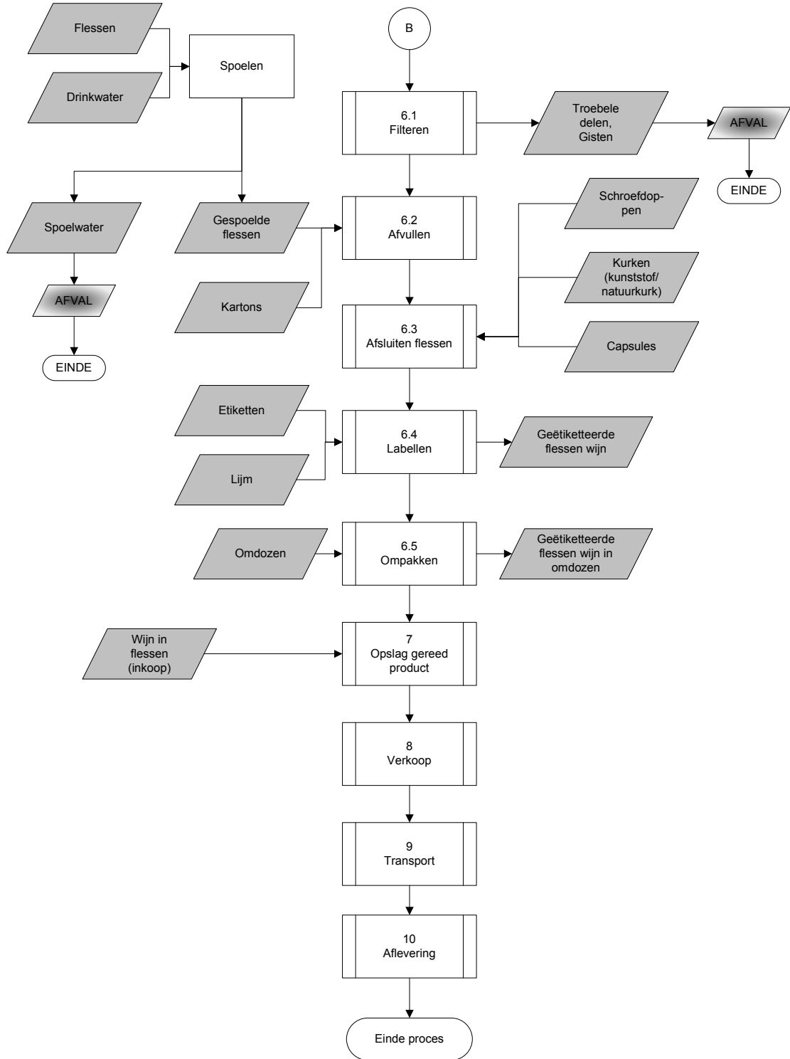
Figuur 7.4: Processchema gedetailleerd III: Bottelen t/m Afleveren
