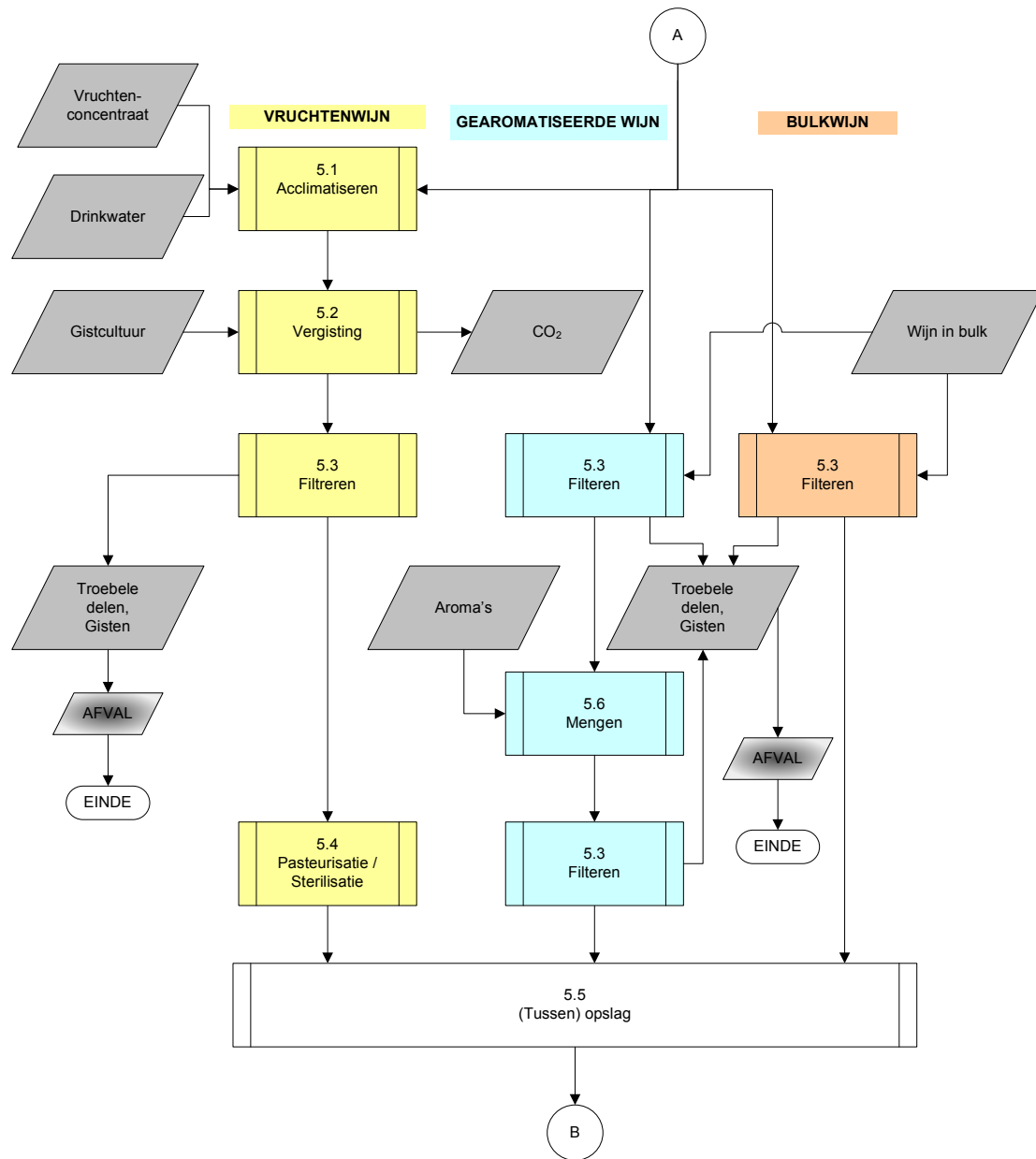
Figuur 7.3: Processchema gedetailleerd II: Verwerking
